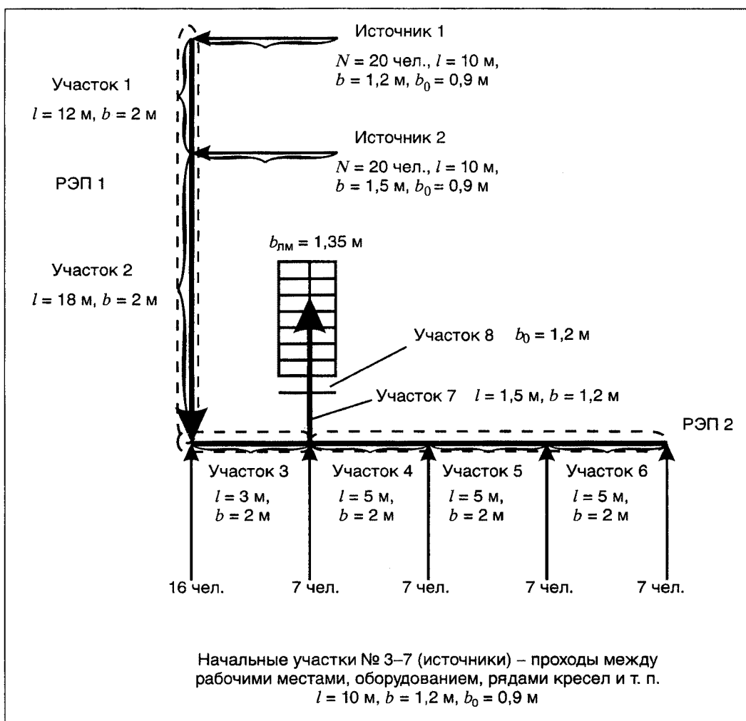
Рис. П5.2. Пример составления расчетной схемы эвакуации людей по части этажа до входа в лестничную клетку:
