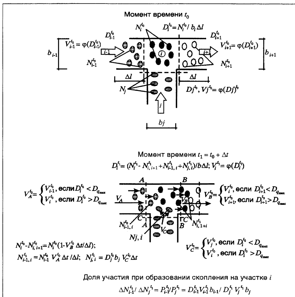
Рис. П4.1. Изменения состояния потока в последовательные моменты времени
