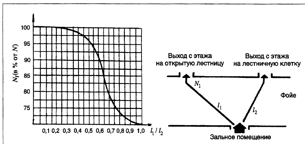
Рис. П5.5, б. Число зрителей, эвакуирующихся по открытой лестнице: N - общее количество эвакуирующихся; N_1 - число эвакуирующихся по открытой лестнице; l_1 - длина пути до открытой
