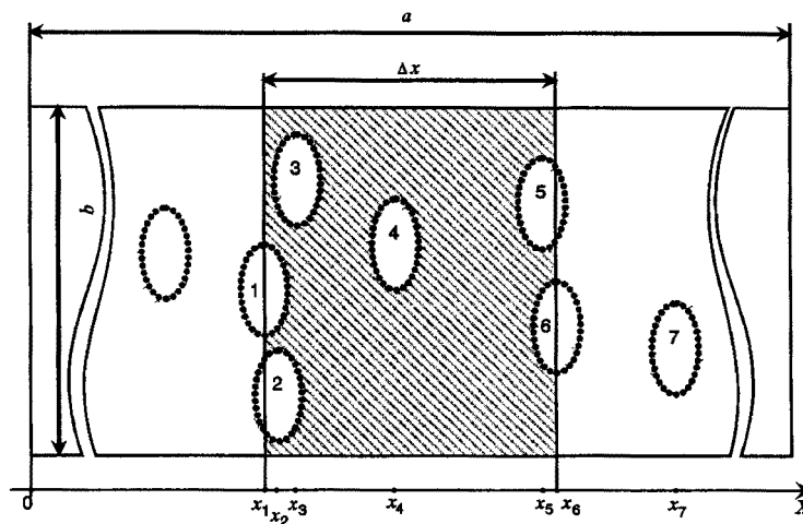
Рис. ПЗ.1. Координатная схема размещения людей на путях эвакуации
