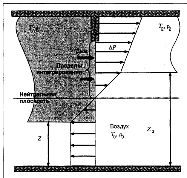
Рис. Пб.1. Массопотоки через проем
